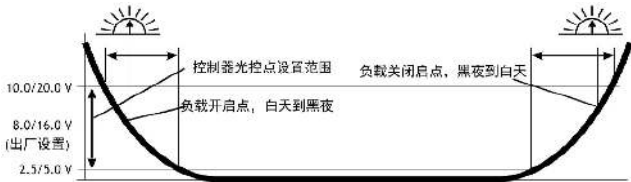
太阳能电池板开路电压曲线
